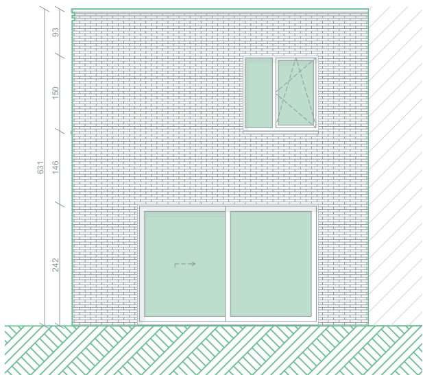
achtergevel
